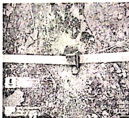
接地扁铁与接地极搭接面不符合规范要求
