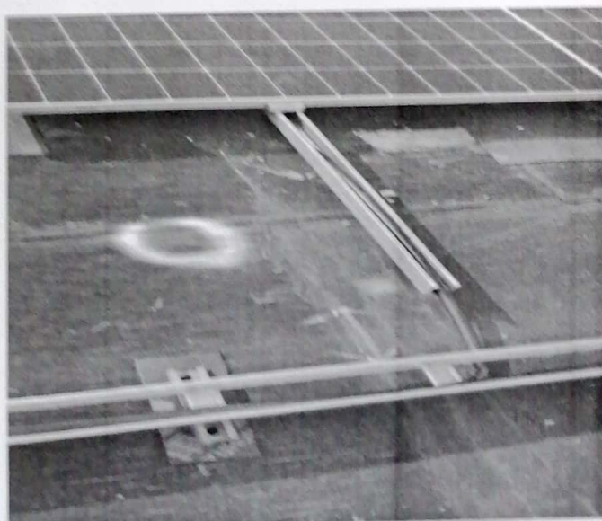
直流线穿管已穿到位无露线 线
