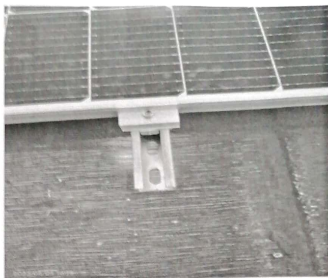
边压穿刺片安装贴合
