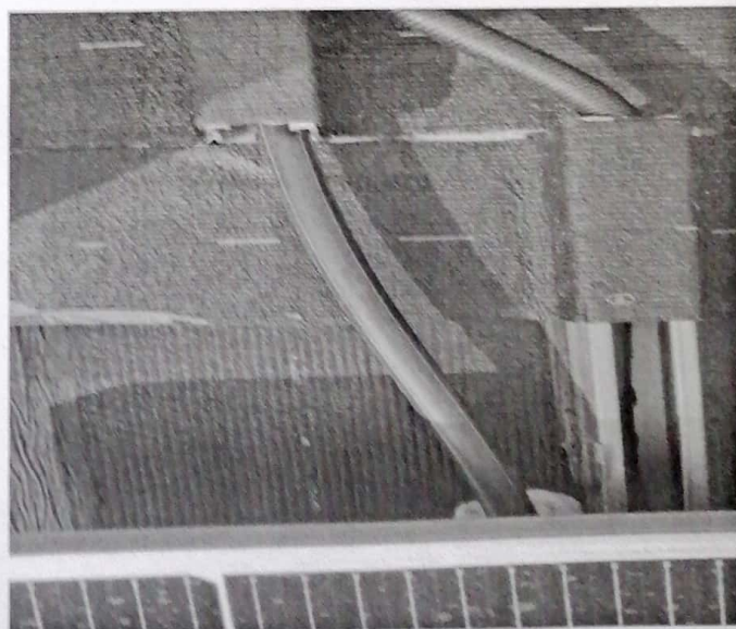
直流线穿管已穿到位无露
