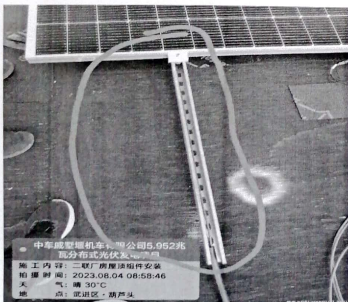
直流线穿管存在没穿到位置露线
