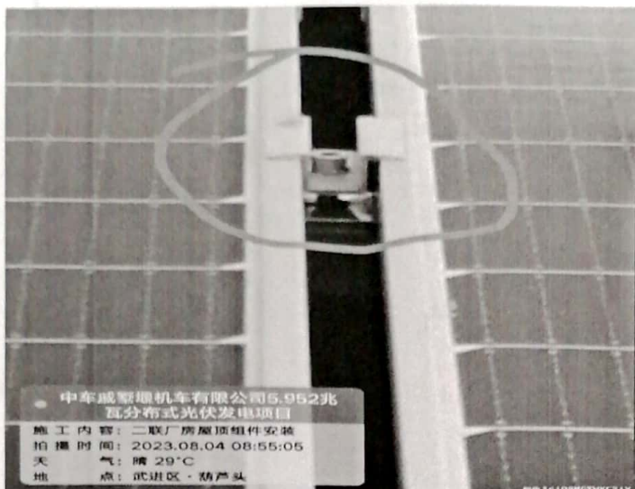
中压块安装不吻合
