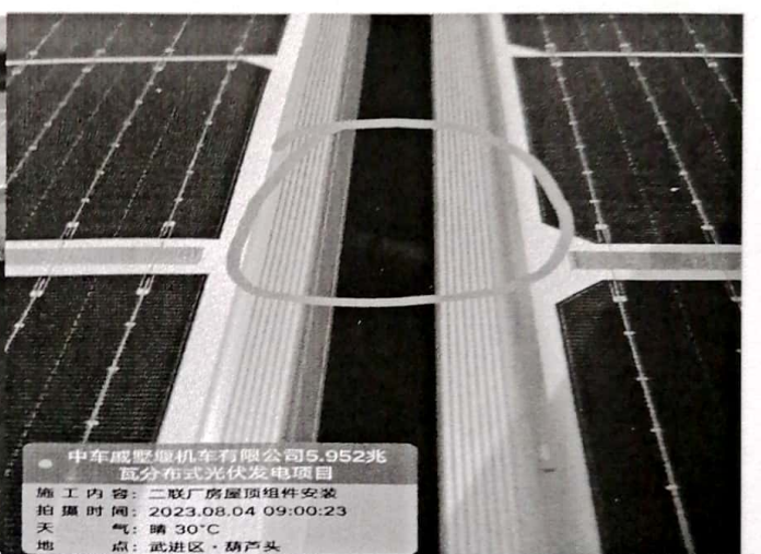
M4 头暴露在组件中压间距中
