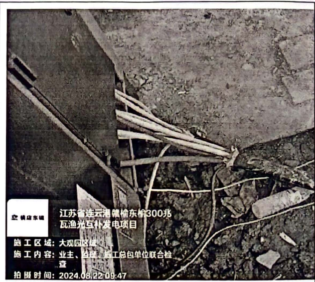
配电柜临时电缆接线不规范
