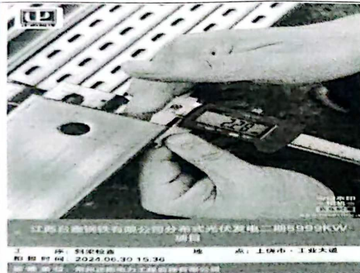
连接件高度与图偏差15mm
