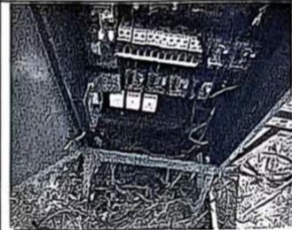
3.配电箱底部未封闭，接线不规范，未张贴负责人及联系方式，线缆走线需避开材料加工区。
