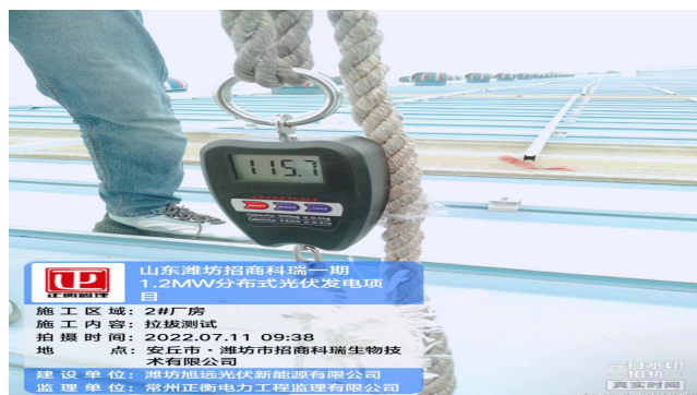
拉拔测试
