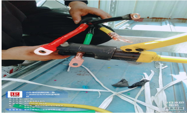
3#厂房电缆头制作
