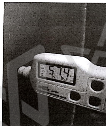
防腐涂层干漆膜厚度不符合设计要求
