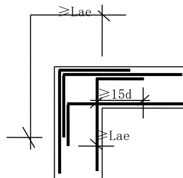
转角接头
