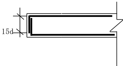
端部无暗柱墙
