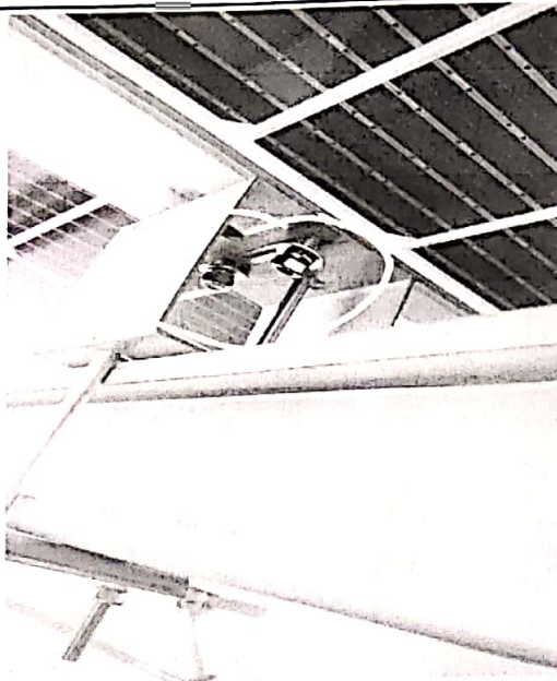
光伏组件连接支架横梁螺栓未紧
