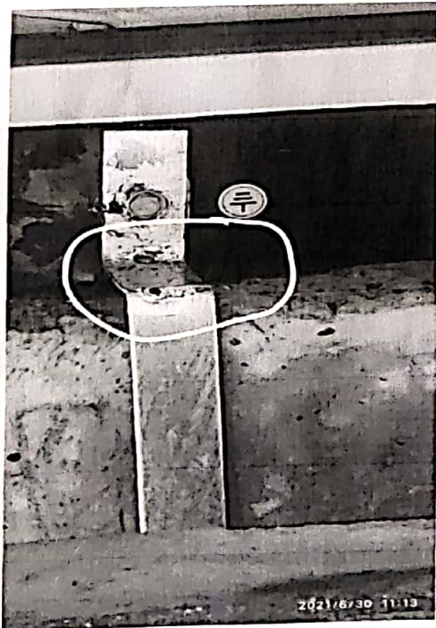
箱变设备接地不符合要求
