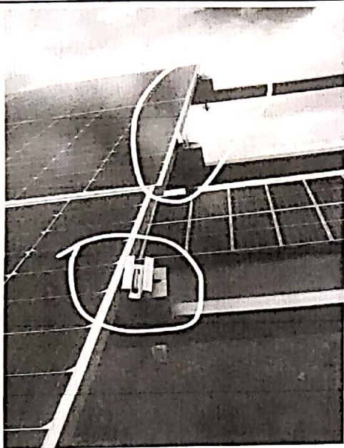
光伏组件边压块安装不符合要求
