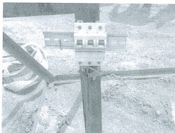
机械设备未设漏电保护器
