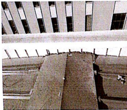
周边过低女儿墙无安全防护栏
