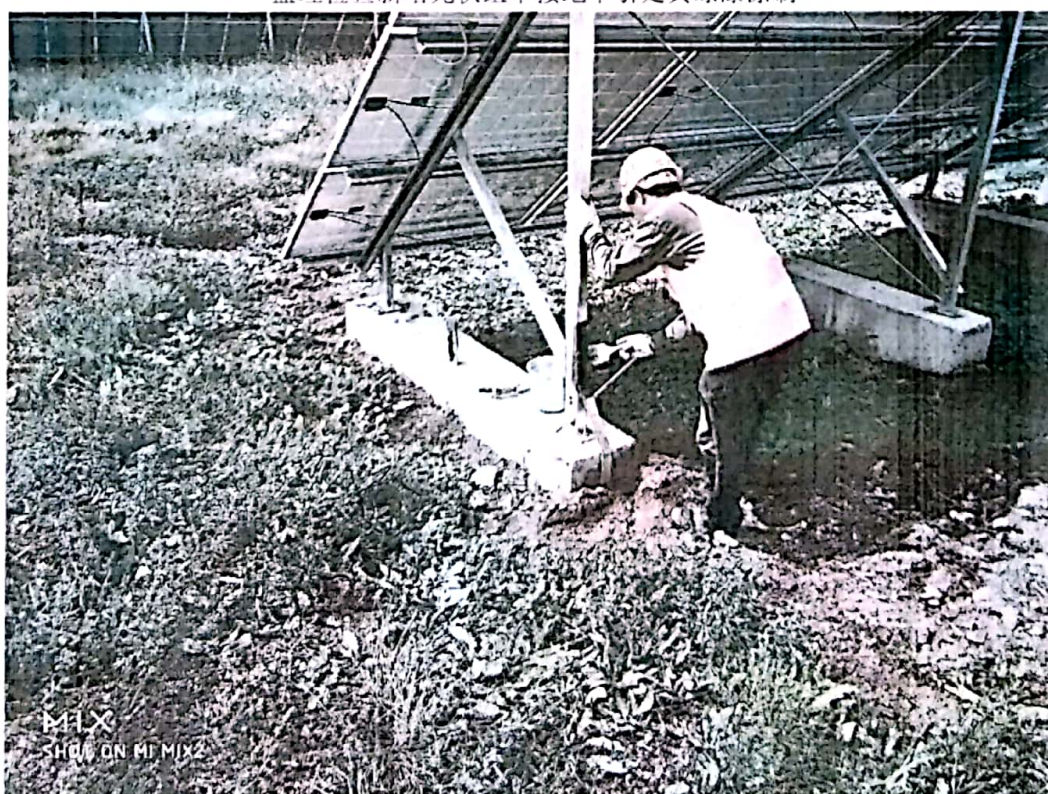
接地下引焊接处防腐处理
