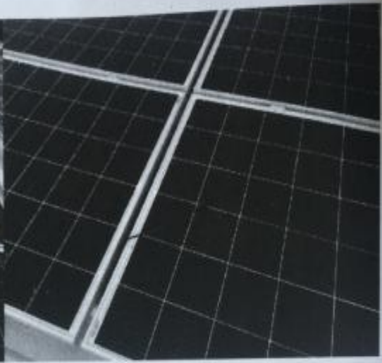
部分组件 MC4 插接头没有防水措施
