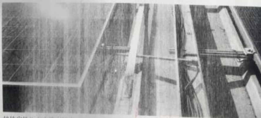
接地扁铁压在电焊网上
