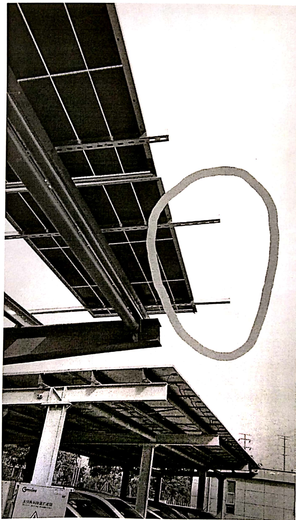
车棚东区后排两根光伏支架长度比设计长度多 20mm
