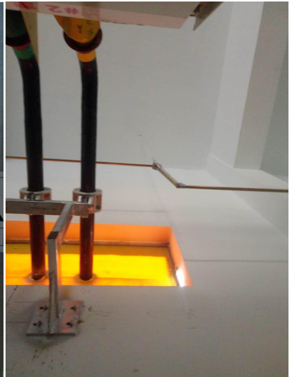
主变低压侧照明管改造
