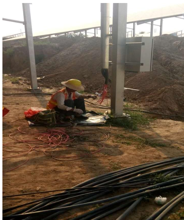
汇流箱接线
