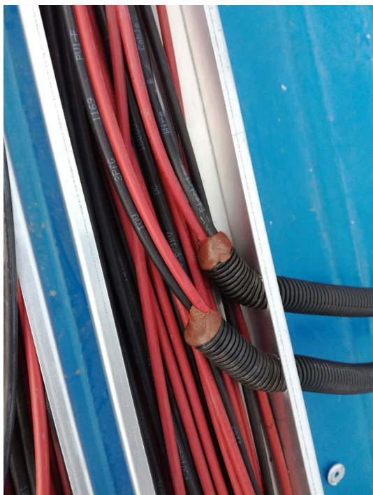
套管封堵
