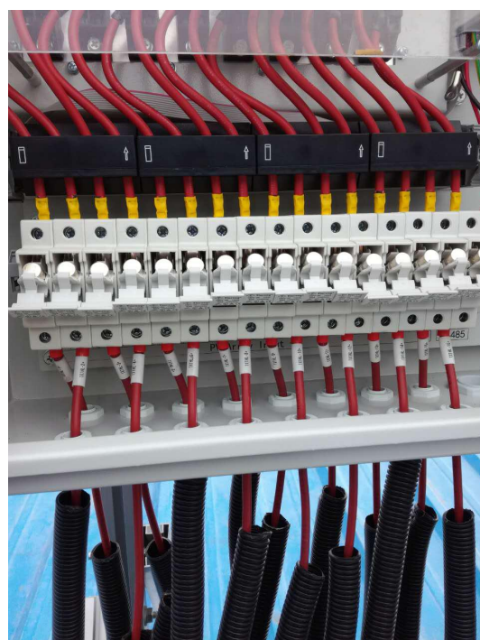
汇流箱接线
