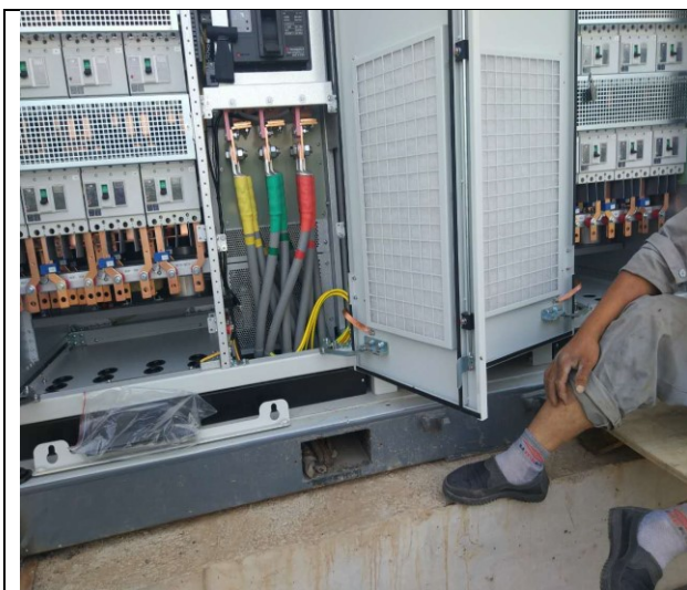
逆变器接线
