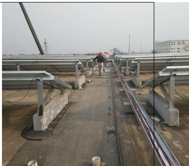
型材主车间直流电缆敷设
