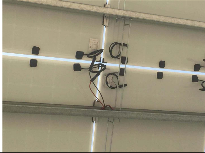
MC4 接头制作
