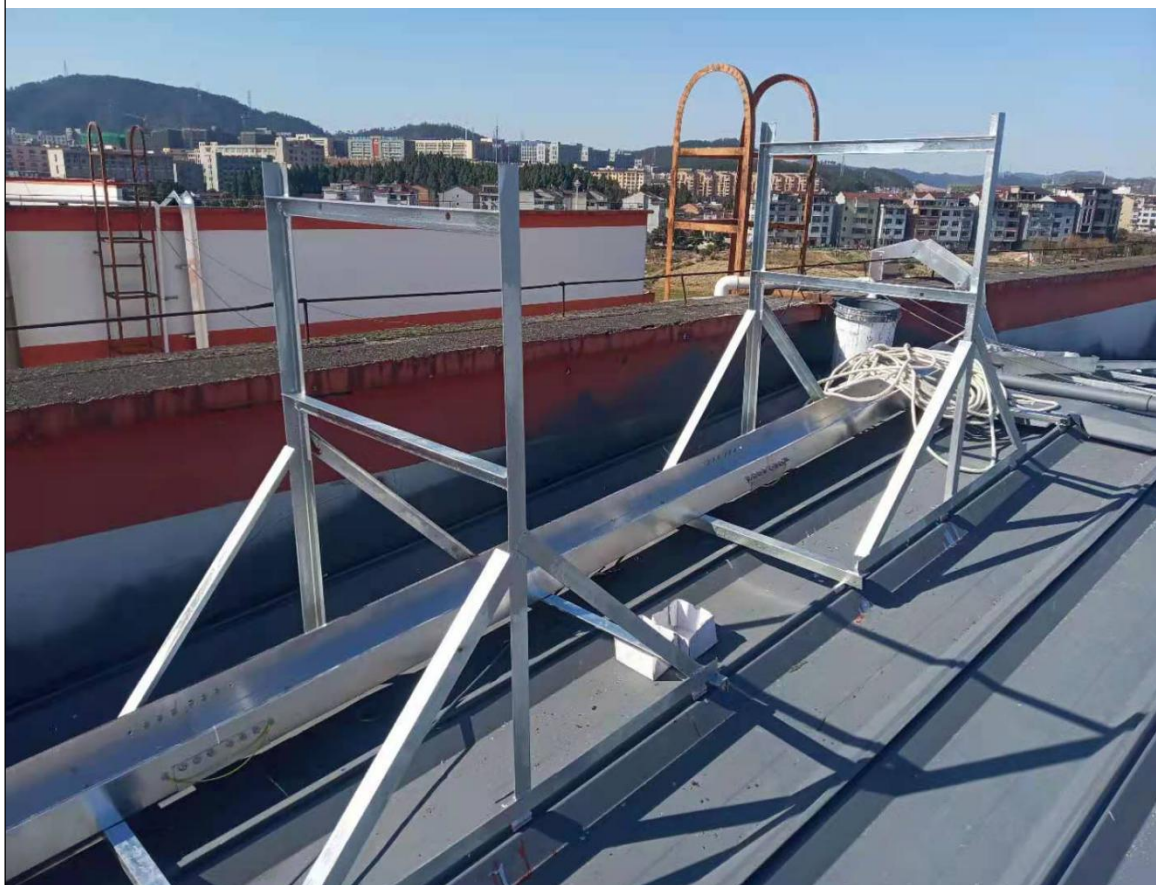
图 4: 铝导轨安装
