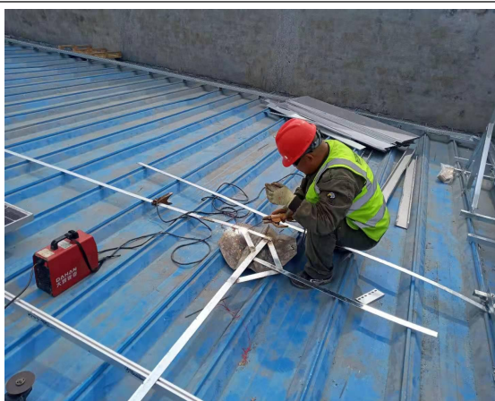
图 3：接地焊接
