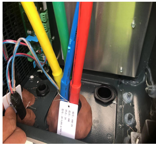
并网柜电缆悬挂标识牌、防火封堵
