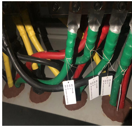
并网柜电缆悬挂标识牌、防火封堵
