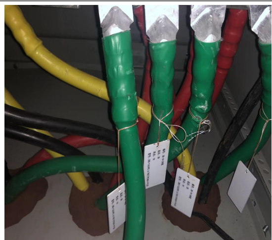
逆变器电缆标识牌安装、防火封堵
