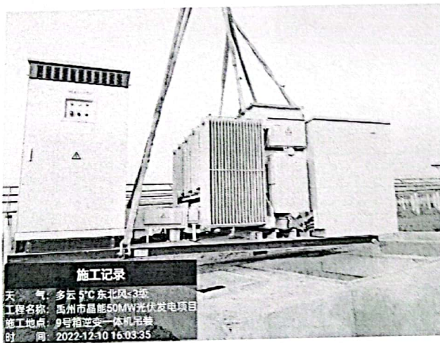
箱逆变一体机吊装就位
