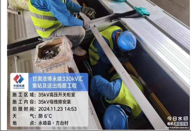
甘肃浩博永靖330kV汇集站及送出线路工程 施工区域: 35kV高压开关柜室 施工内容: 35kV母线排安装 拍摄时间: 2024.11.23 14:53 天气: 阴 6°C 地点: 永靖县·方台村
