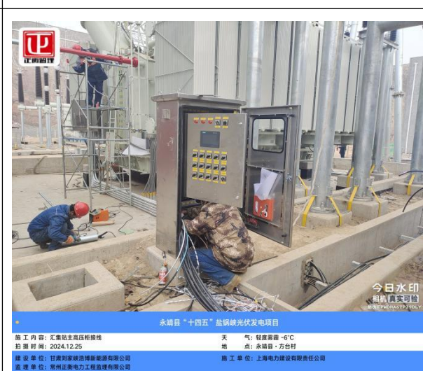
永靖县“十四五”盐锅峡光伏发电项目 施工内容: 汇集站主变高压柜接线 天气: 轻度雾霾 -6℃ 拍摄时间: 2024.12.25 地点: 永靖县·方台村 建设单位: 甘肃刘家峡清洁能源有限公司 监理单位: 常州正泰电力工程监理有限公司 施工单位: 上海电力建设有限责任公司
