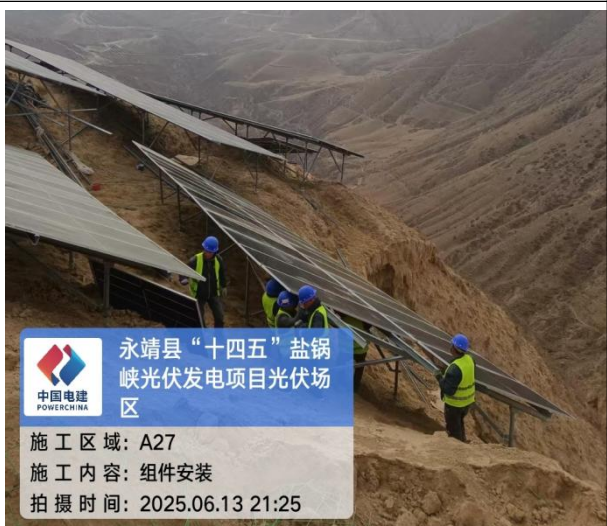
组件安装
