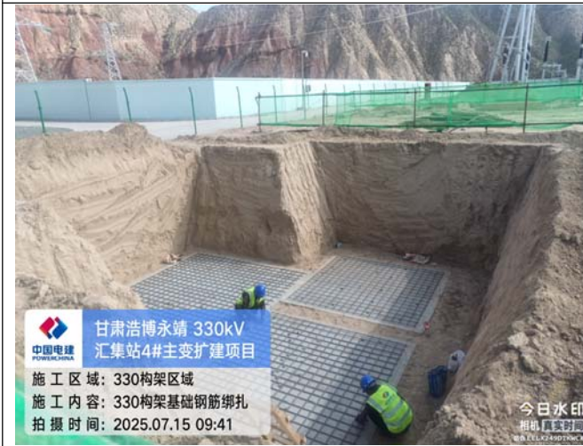
构架基础钢筋绑扎
