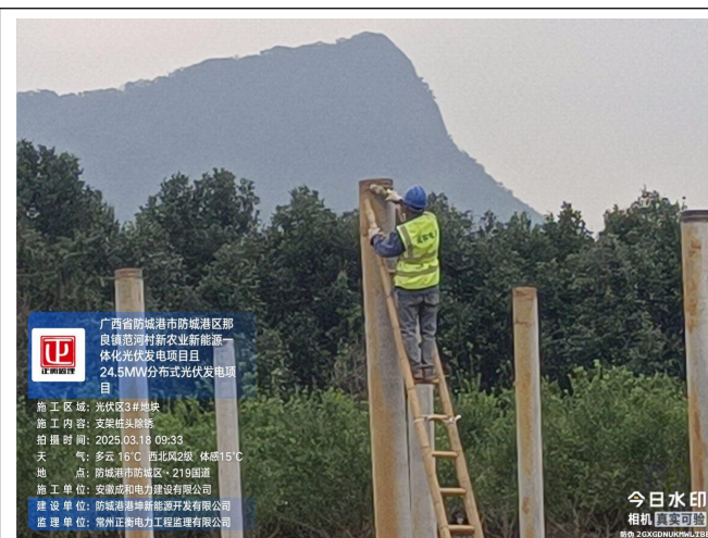
监理巡查三地块支架桩头除锈
