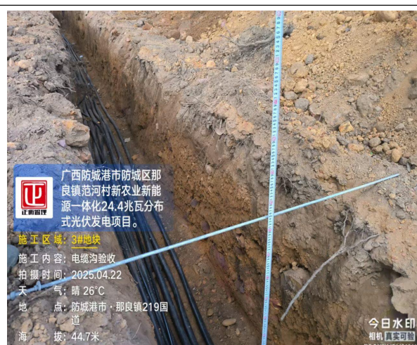
监理巡查光伏区三号地块电缆沟验收
