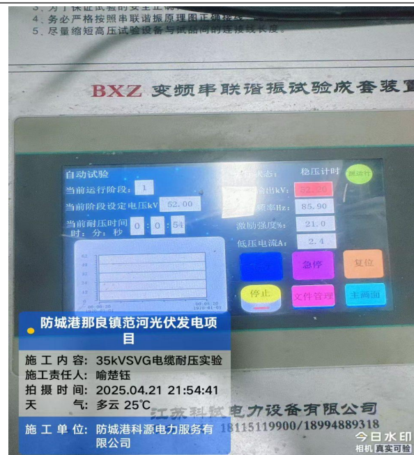
监理巡查光伏区升压站 35KV 电缆耐压试验
