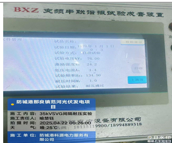
监理巡查光伏区升压站 35KV 隔离耐压试验
