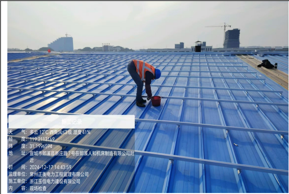
导轨安装
