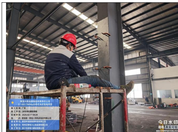
2#车间加固柱脚贴板安装
