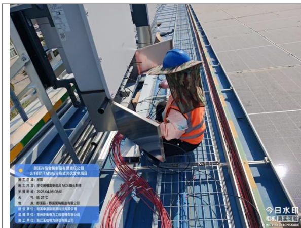
逆变器槽盒安装及 MC4 插头安装
