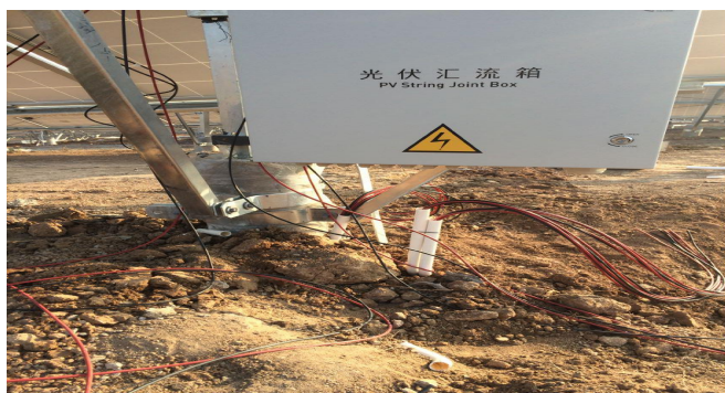
4、1*4 电缆穿管预埋深度不符合设计要求
