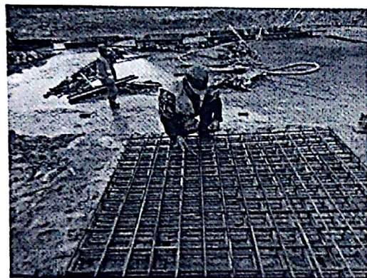
配电房基础承台钢筋加工
