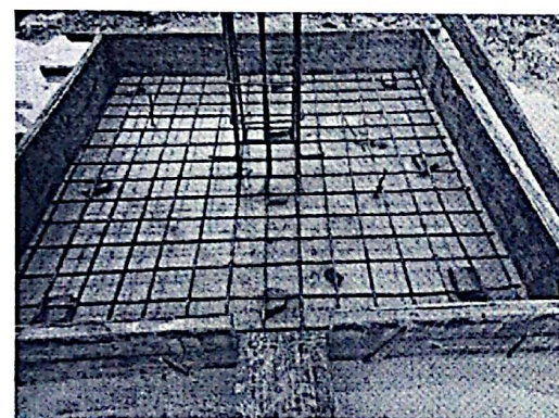
配电房基础承台钢筋隐蔽
