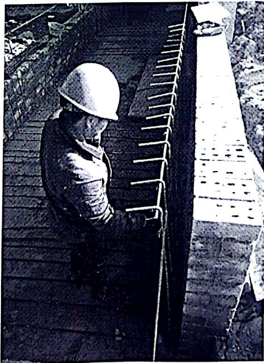
配电房电缆沟钢筋绑扎
