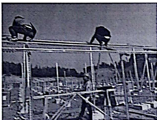
光伏区支架安装
