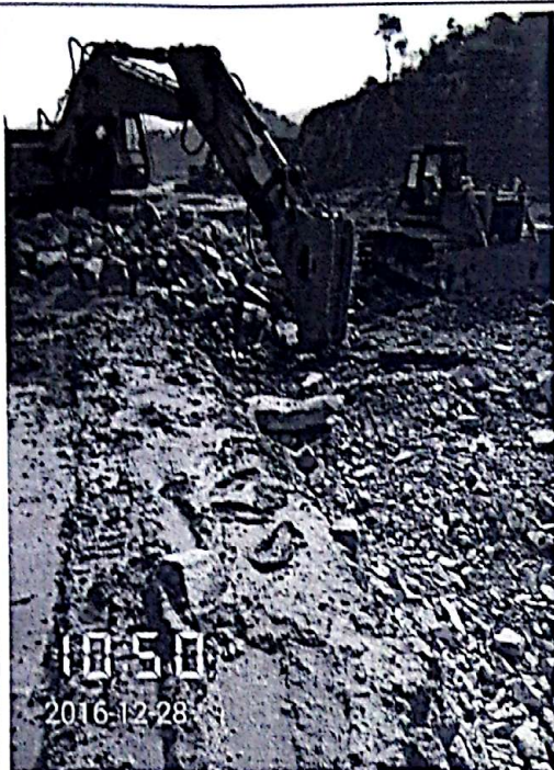
光伏区 8#方阵箱逆变基 础开槽
