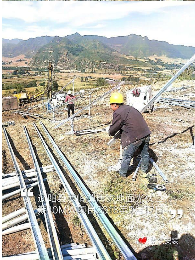
支架安装
