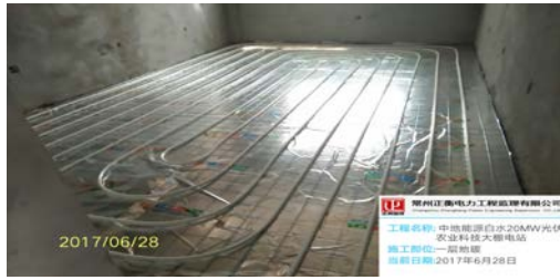
综合楼地暖施工
