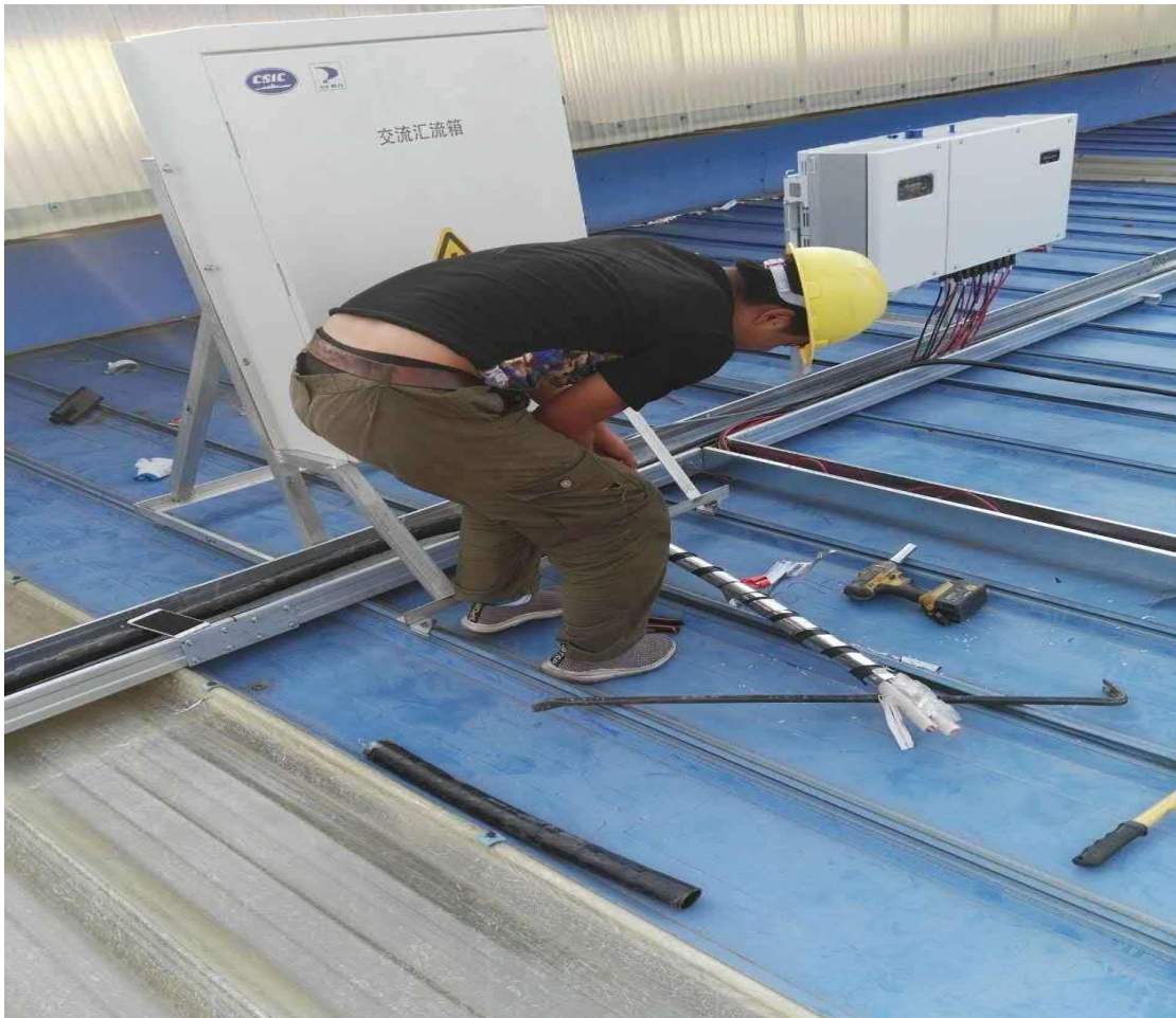
汇流箱施工
