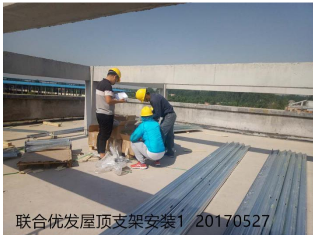
联合优发屋面安装支架20170526
