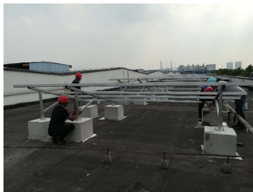
03 混凝土屋面组件支架基础工程
