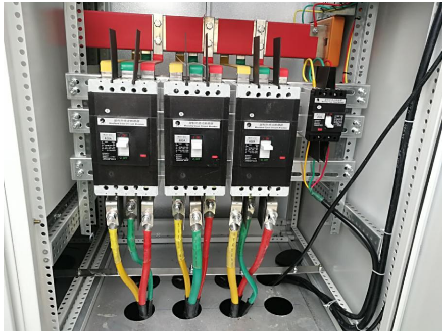
誉丰箱变低压接线完成
