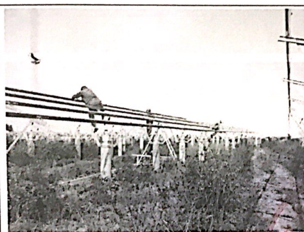
24 区支架安装
