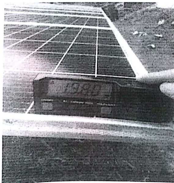
倾角度检查
