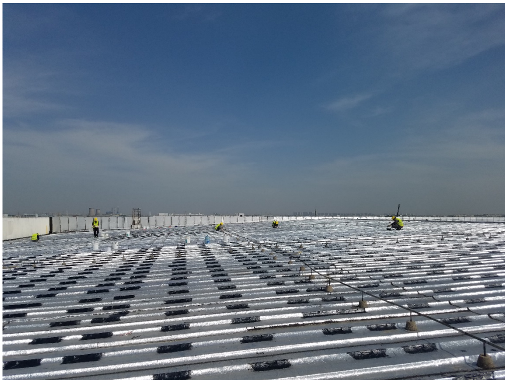
201 车间屋面夹具基础整体施工情况
