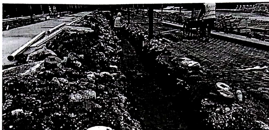
电缆沟垫层铺沙及镀锌管焊接
