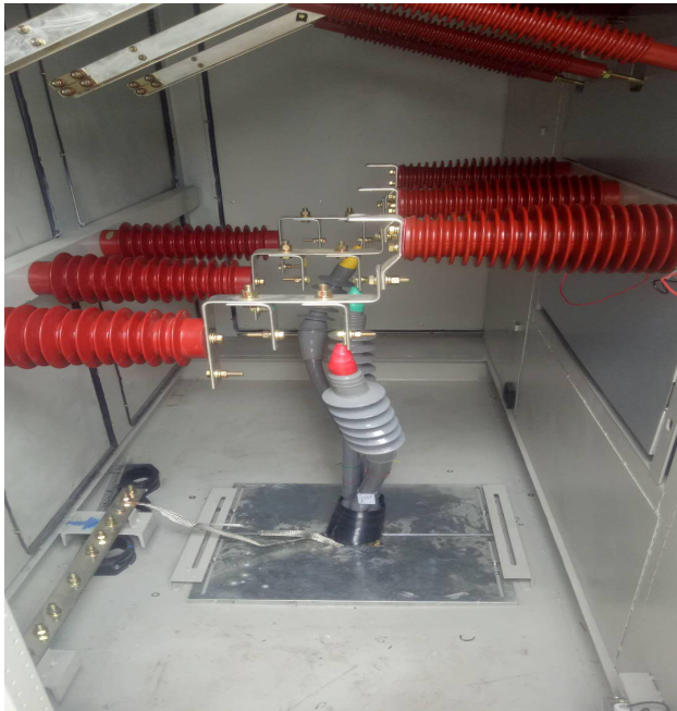
高压电缆头制作安装完成
